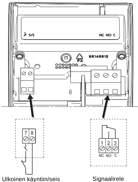
Kuva 1 Liitäntänavat
