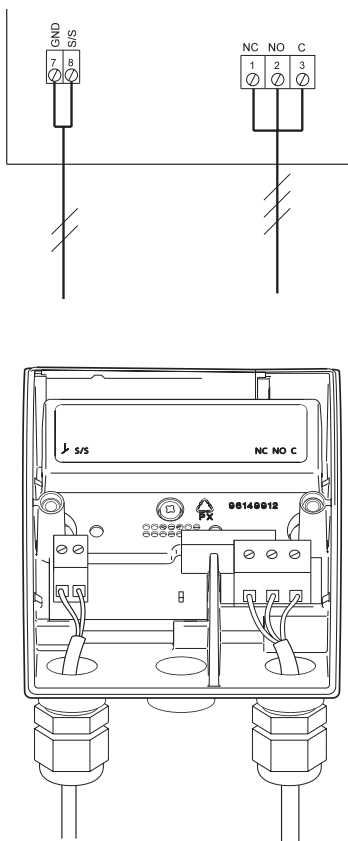
Фиг. 2 Свързване на кабелите
