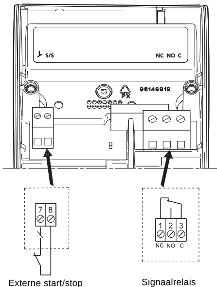
Afb. 1 Aansluitklemmen
