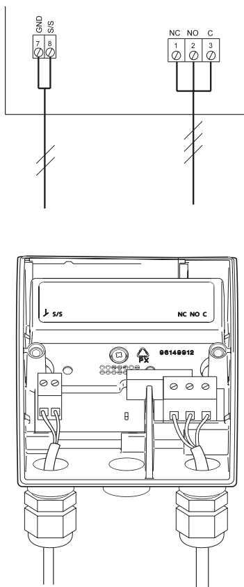
Obr. 2 Připojení kabelu
