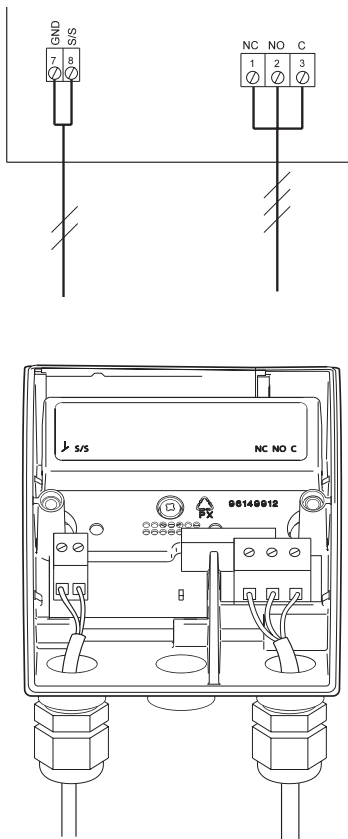
Joonis 2 Kaablite ühendamine
