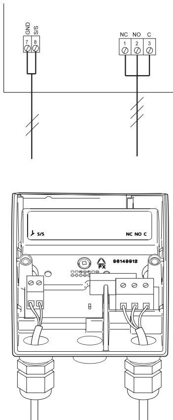
Fig. 2 Kabelanslutning
