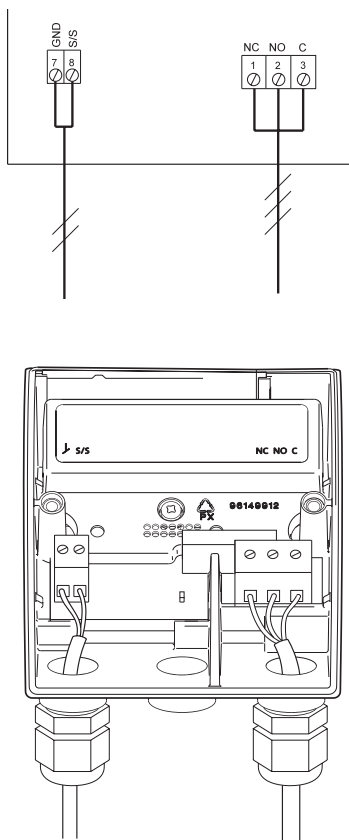
Slika 2 Kabelski spoj
