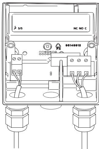
Skica 2 Priključitev kablov
