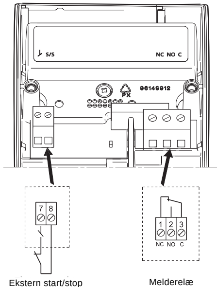
Fig. 1 Tilslutningsklemmer
