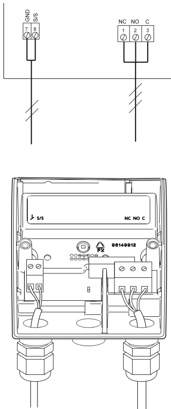
Şekil 2 Kablo bağlantısı
