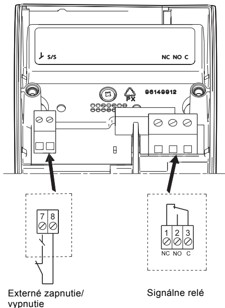
Obr. 1 Pripájacie svorky
