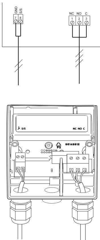
2 pav. Kabelių jungtys
