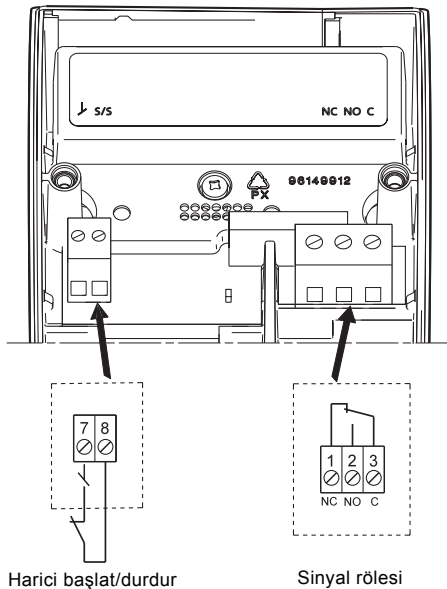
Şekil 1 Bağlantı terminalleri
