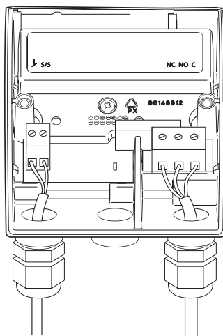
Afb. 2 Kabelaansluiting
